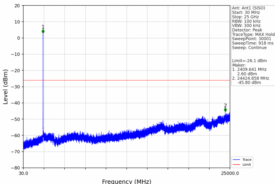
802.11b_LCH_2412MHz_Ant1 (SISO)_NTNV
