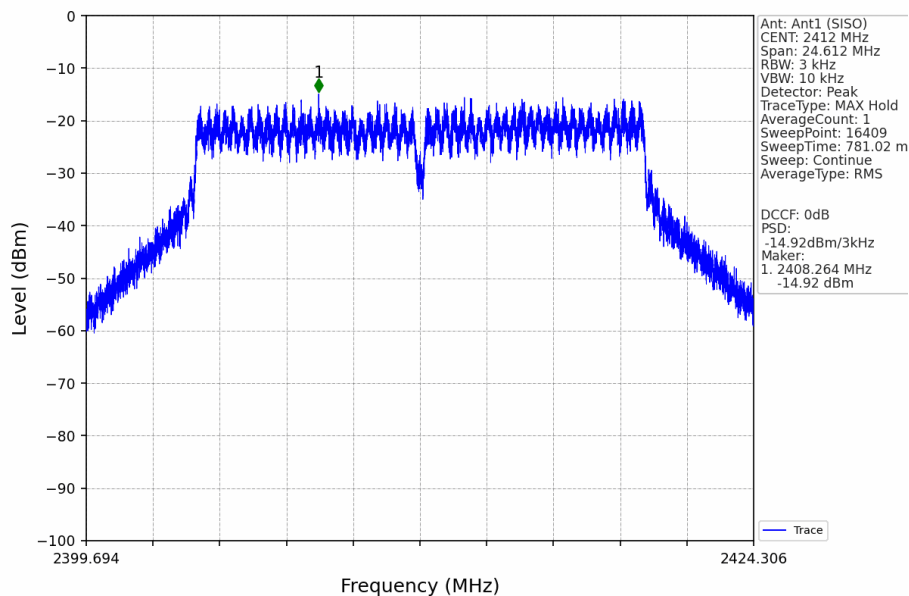
802.11g_LCH_2412MHz_Ant1 (SISO)_NTNV
