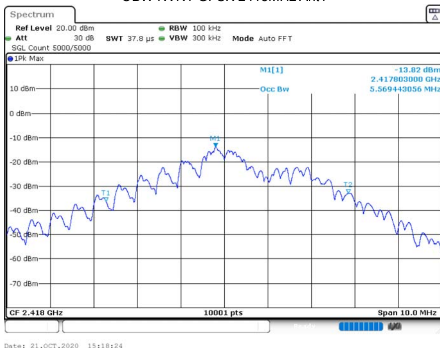
OBW NVNT GFSK 2418MHz Ant1
