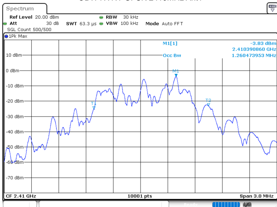
OBW NVNT GFSK 2410MHz Ant1
