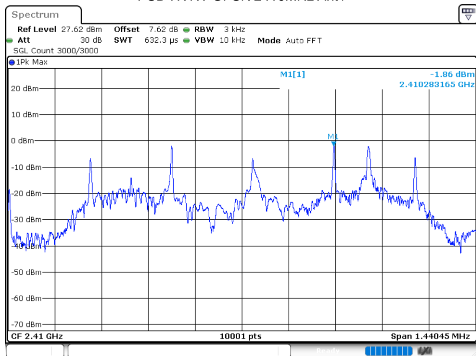
PSD NVNT GFSK 2410MHz Ant1
