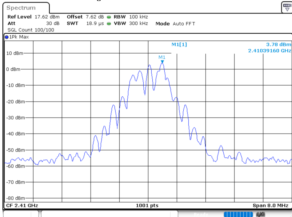
Band Edge NVNT GFSK 2410MHz Ant1 Ref
