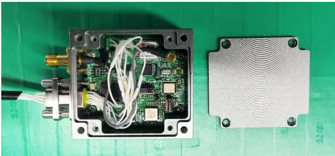
(40) EUT Photo
