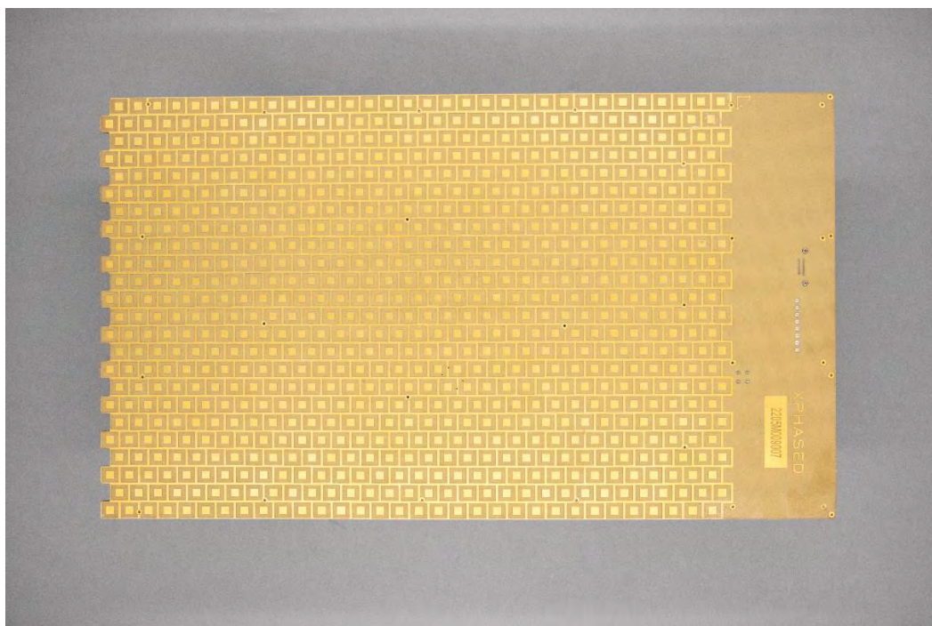
(13) EUT Photo
