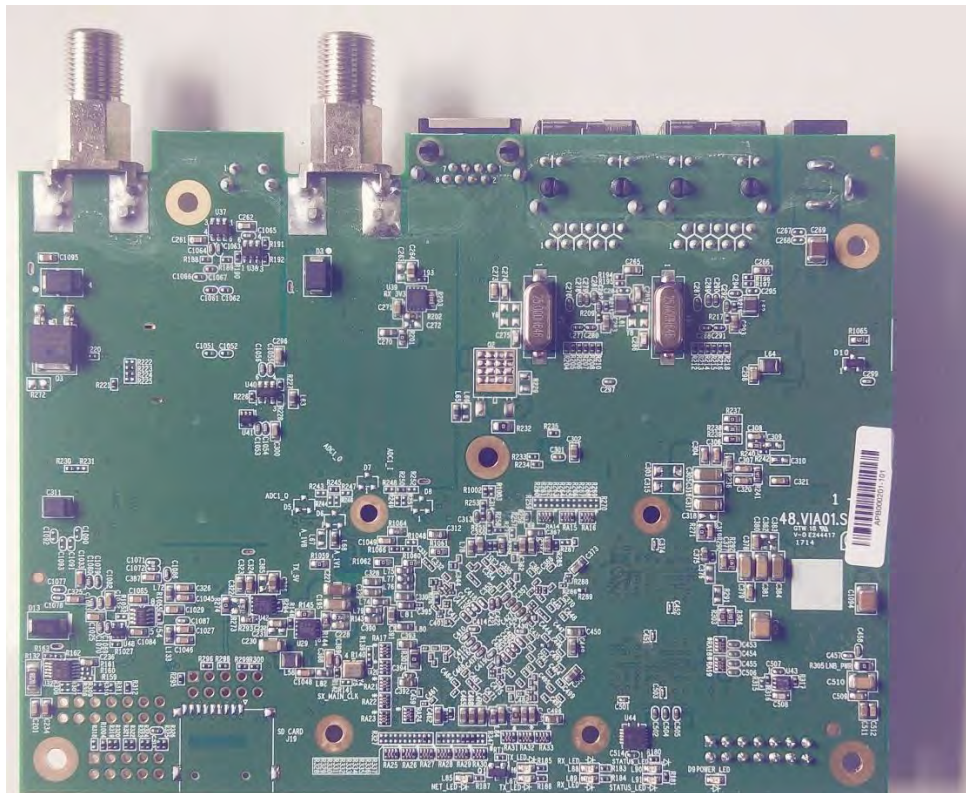
(20) EUT Photo
