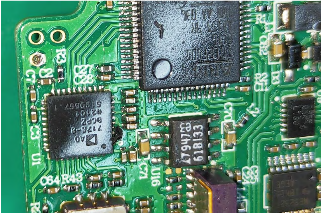
(46) EUT Photo
