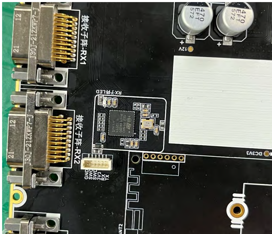
(10) EUT Photo
