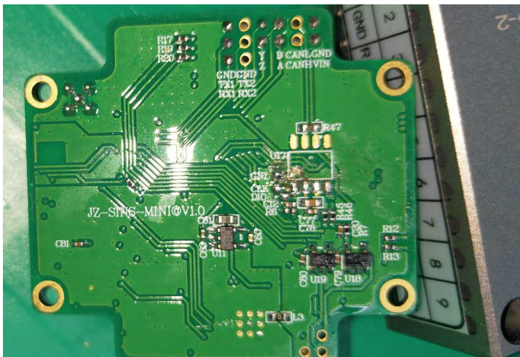
(46) EUT Photo
