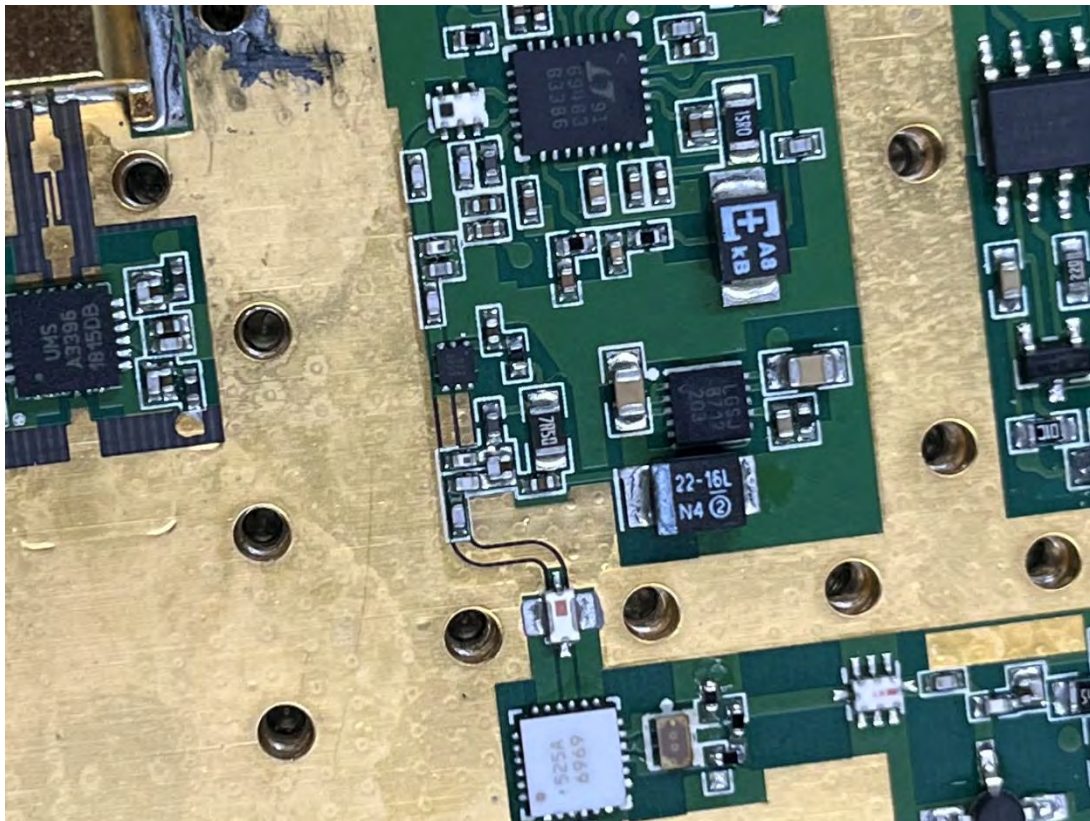
(30) EUT Photo
