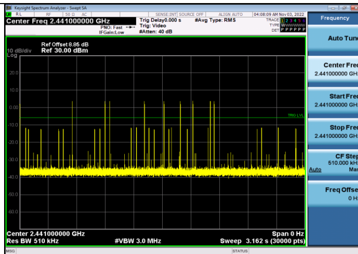
3DH1_Ant1_Hop
