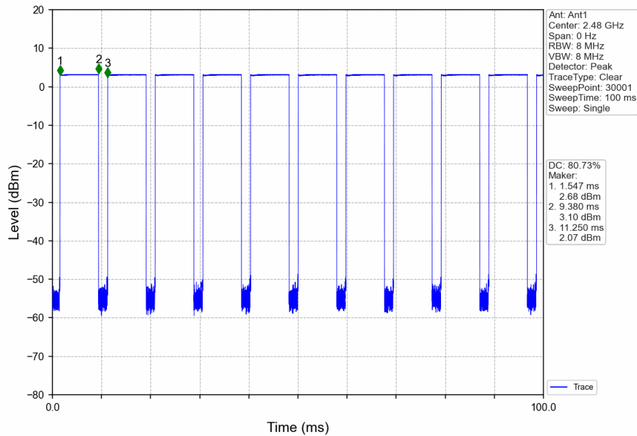
1M_HCH_2480MHz_DataRate=_Ant1_NTNV
