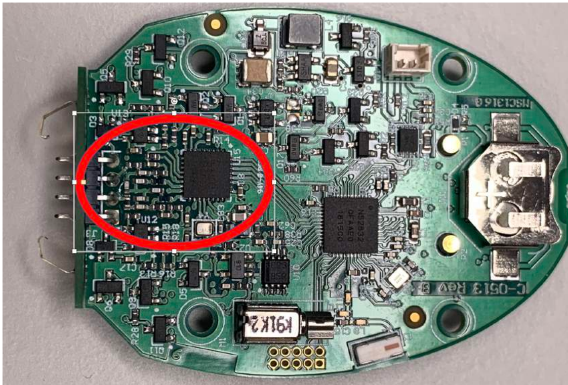
RFID antenna
