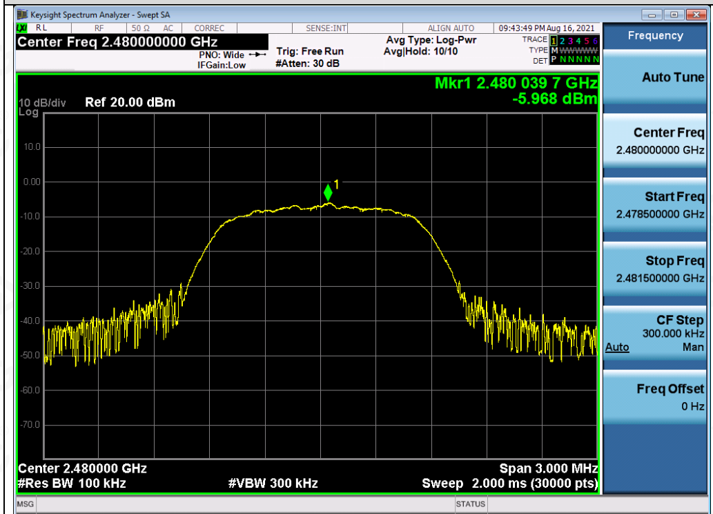
Test_Graph_EDR_ANT1_2480_2Mbps_Reference Level
