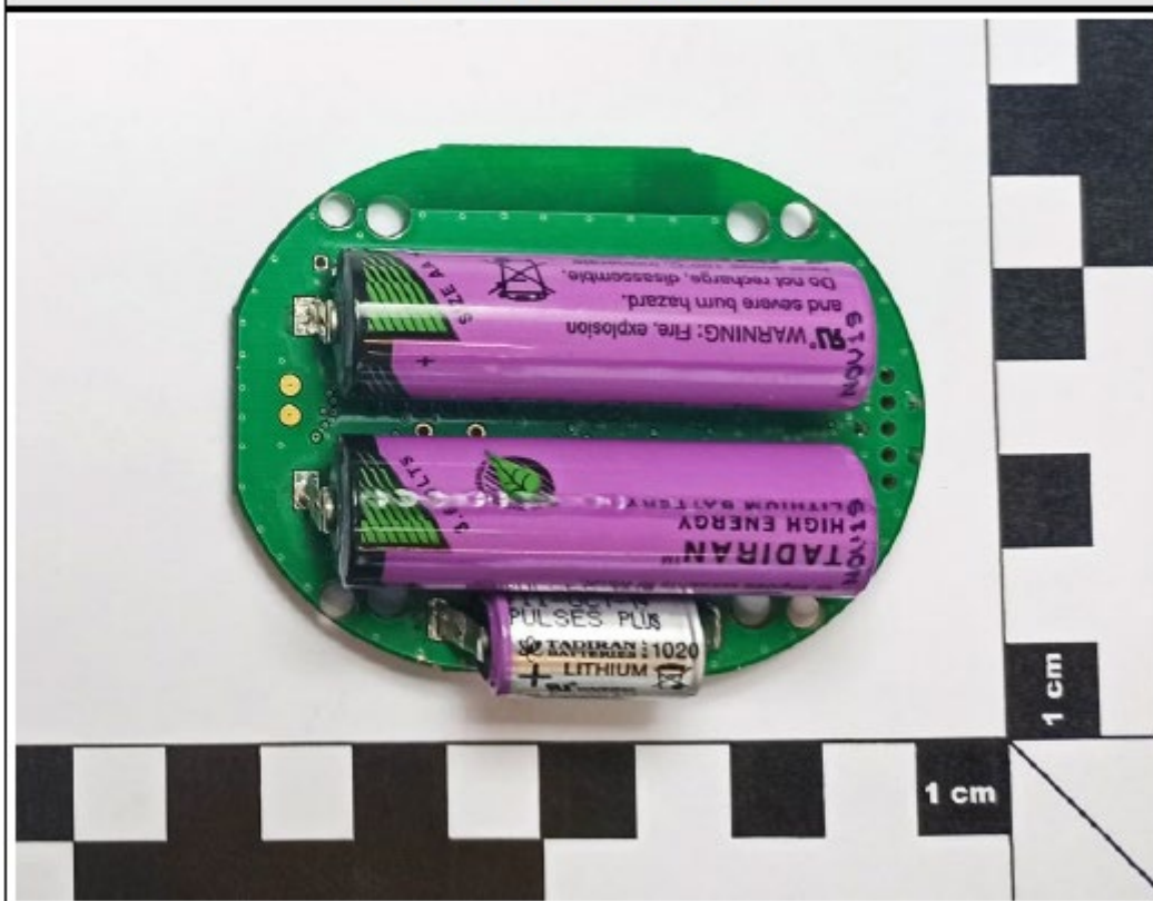
EUT PCB BOTTOM SIDE
