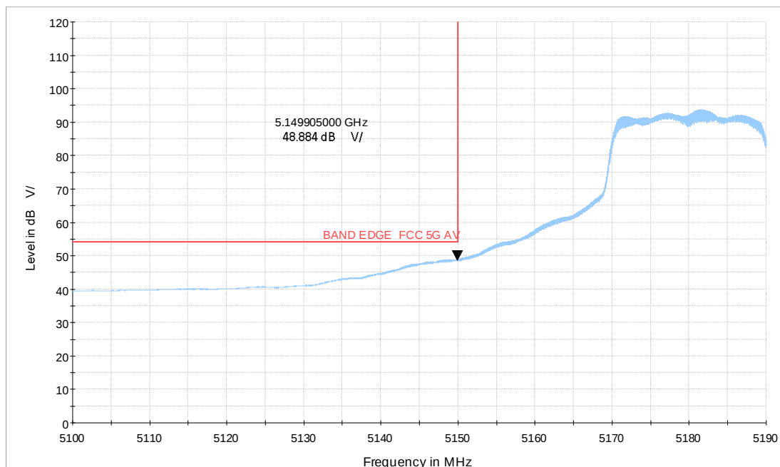
Wi-Fi 5G_ax20 CH36_5.1-5.19GHz_MCS0_MIMO_V_TP22_AV
