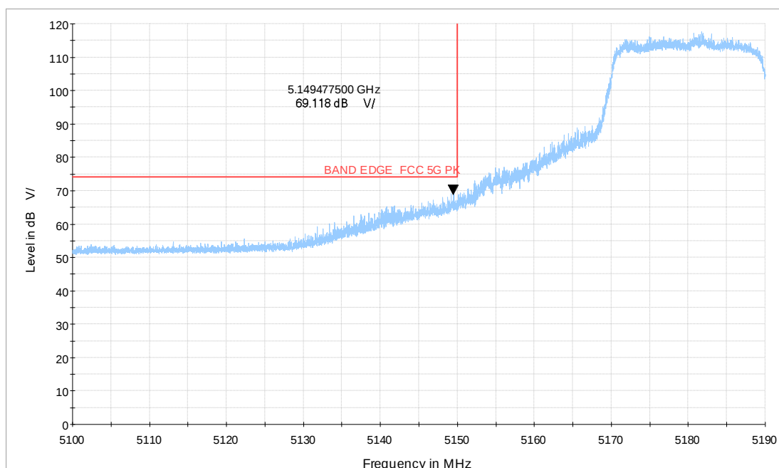
Wi-Fi 5G_ax20 CH36_5.1-5.19GHz_MCS0_MIMO_V_TP22_PK
