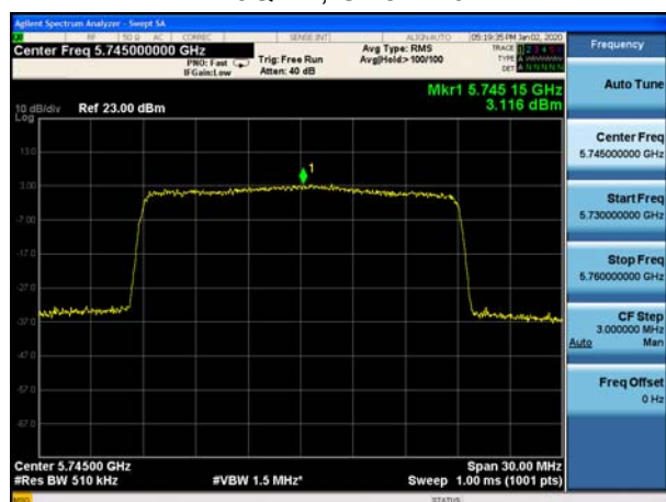
16QAM, CH53140
