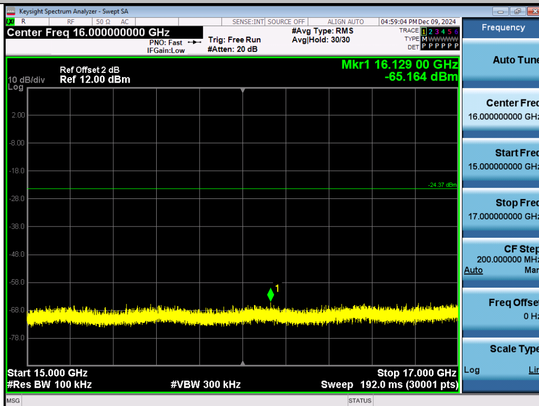
11G-Ant1-2462-15000~17000-PASS
