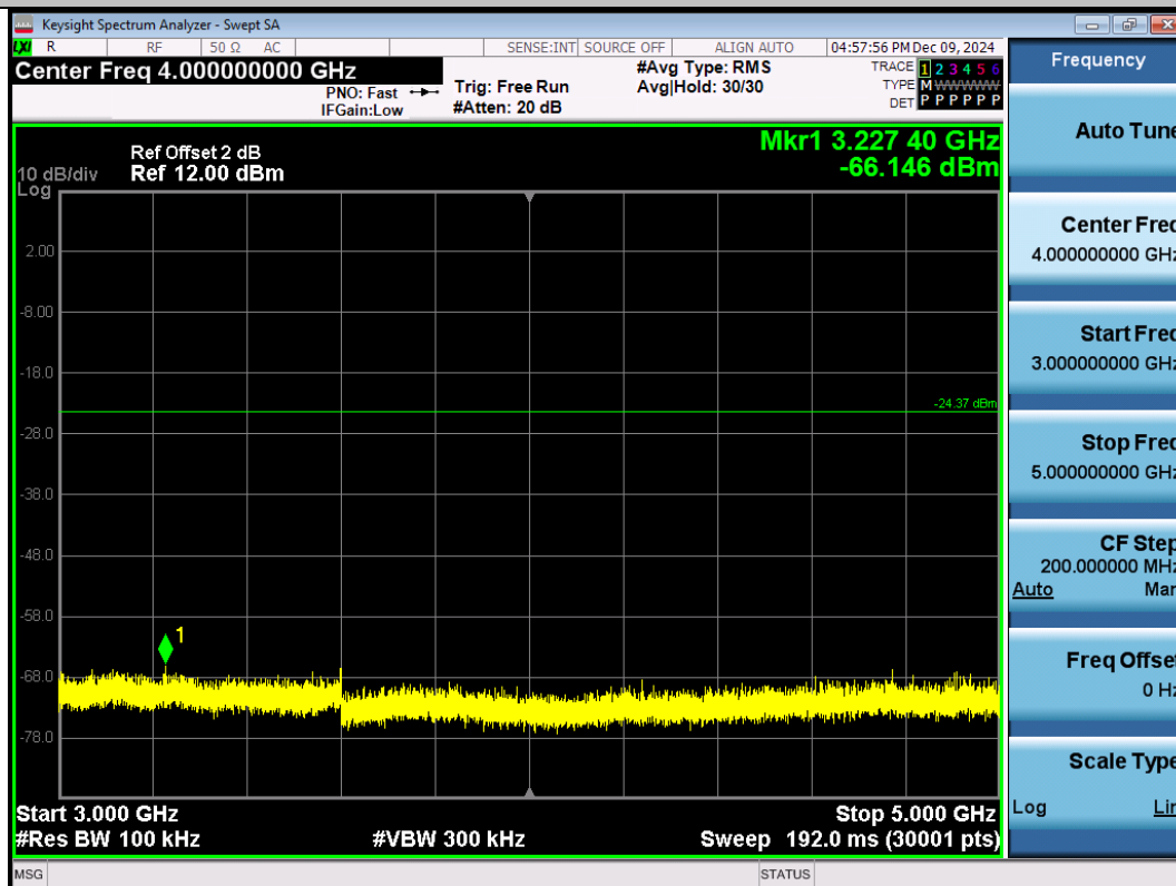
11G-Ant1-2462-3000~5000-PASS
