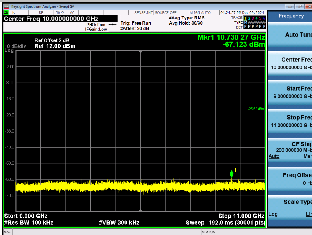
11G-Ant1-2437-9000~11000-PASS
