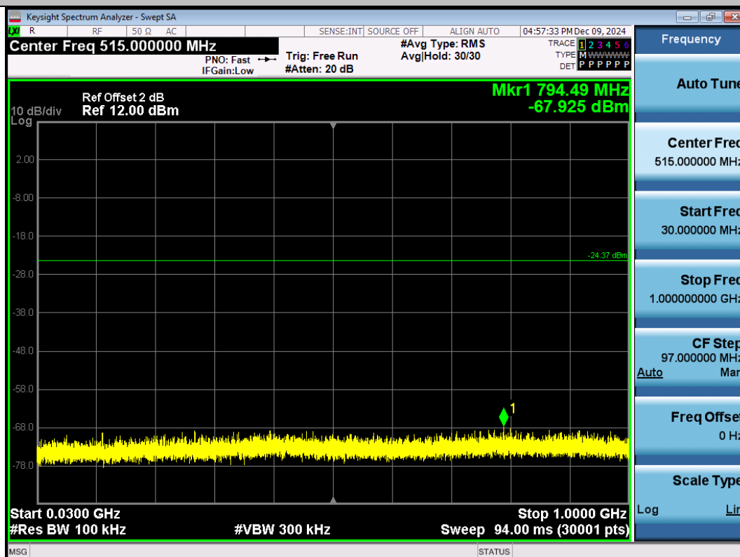
11G-Ant1-2462-30~1000-PASS
