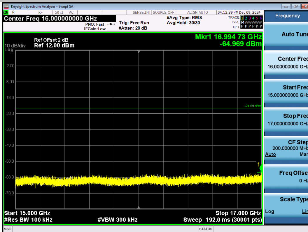
11G-Ant1-2412-15000~17000-PASS
