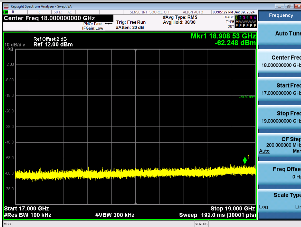
11B-Ant1-2412-17000~19000-PASS
