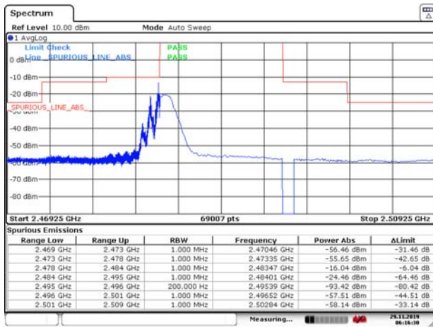
LTE Band 53 1.4MHz QPSK 1RB CH-Low
