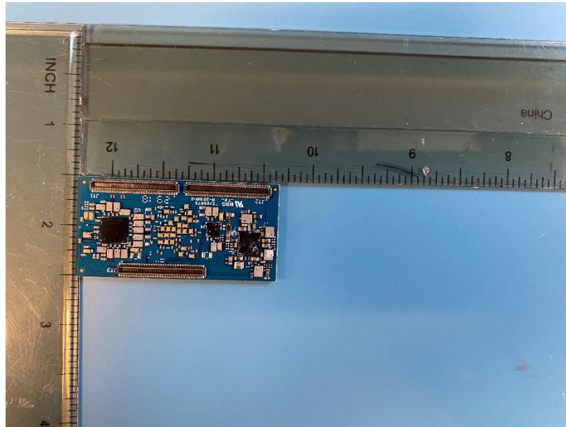
Figure 7: Backside of \mu SOM board
