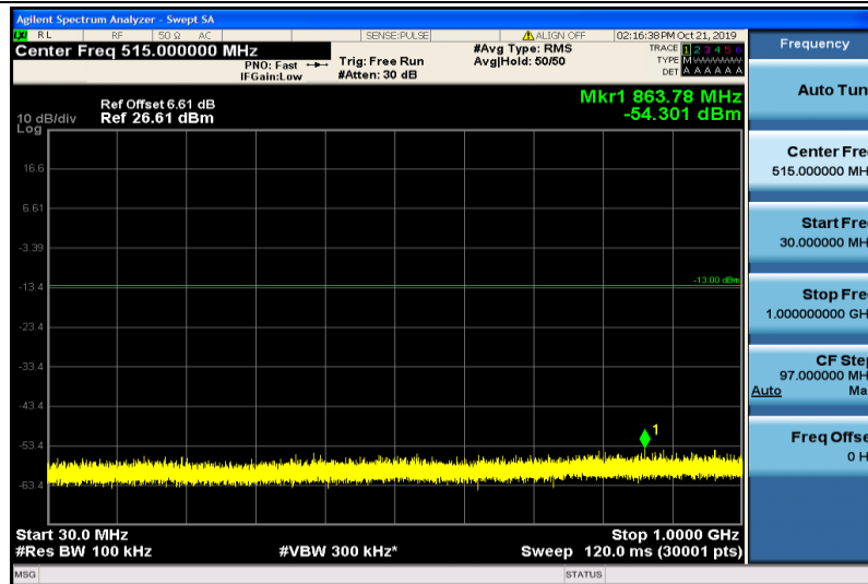
Band4-10MHz-QPSK-20000-1RB#0-30~1000MHz
