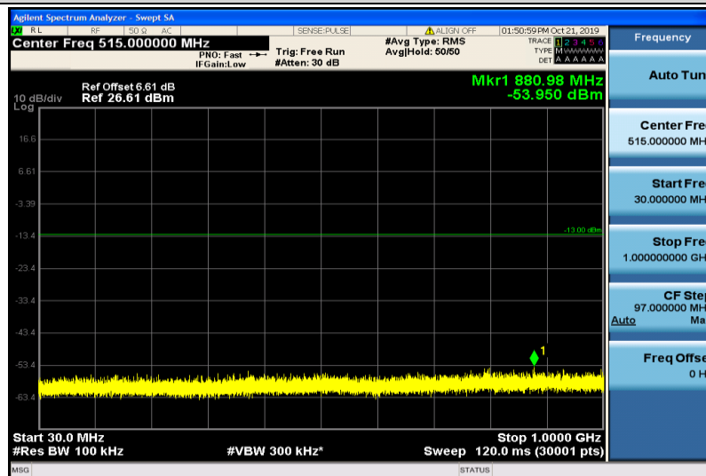
Band4-5MHz-QPSK-20375-1RB#0-30~1000MHz
