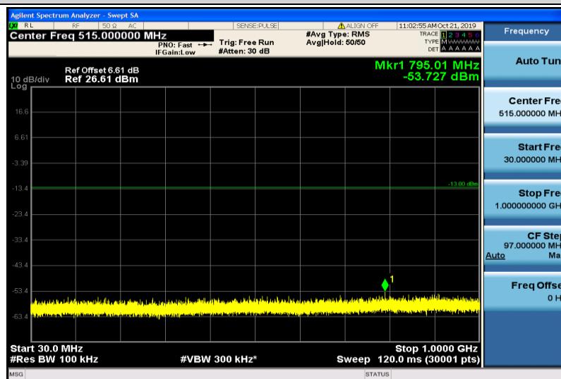
Band4-1.4MHz-QPSK-20393-1RB#0-30~1000MHz
