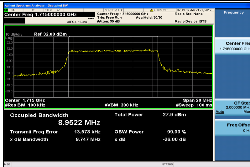
Band4-10MHz-QPSK-20000-50RB#0-8.9522
