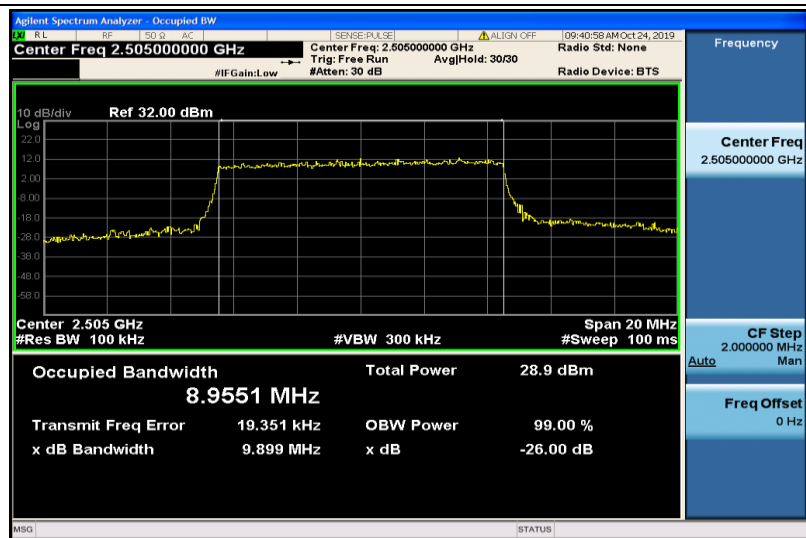
Band7-10MHz-QPSK-20800-50RB#0-8.9551
