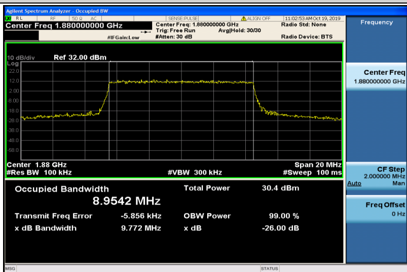
Band2-10MHz-16QAM-18900-50RB#0-8.9542
