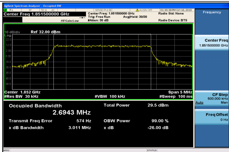
Band2-3MHz-QPSK-18615-15RB#0-2.6943
