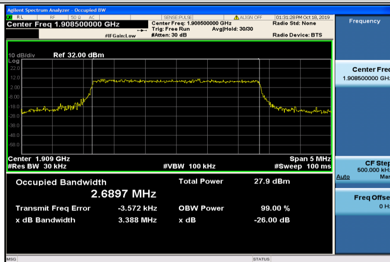
Band2-3MHz-16QAM-19185-15RB#0-2.6897
