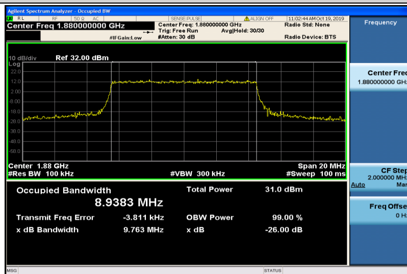
Band2-10MHz-QPSK-18900-50RB#0-8.9383
