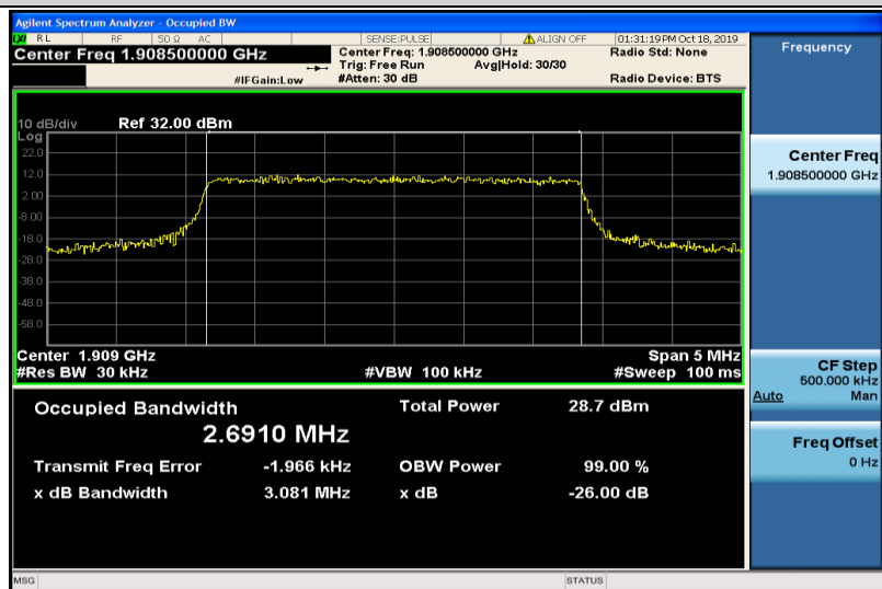
Band2-3MHz-QPSK-19185-15RB#0-2.6910
