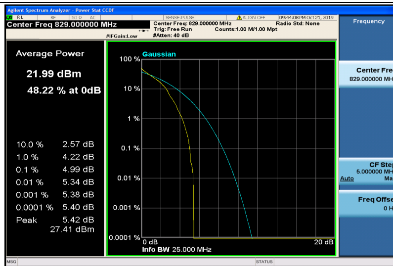
Band5-10MHz-QPSK-20450-1RB#0
