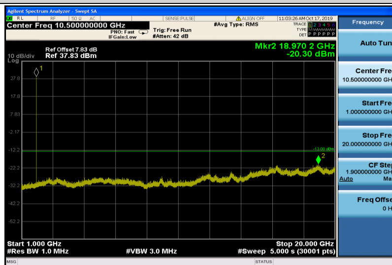
GSM1900-810-1000~20000
