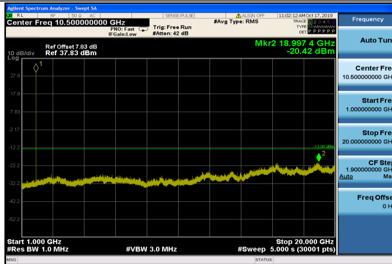
GSM1900-661-1000~20000
