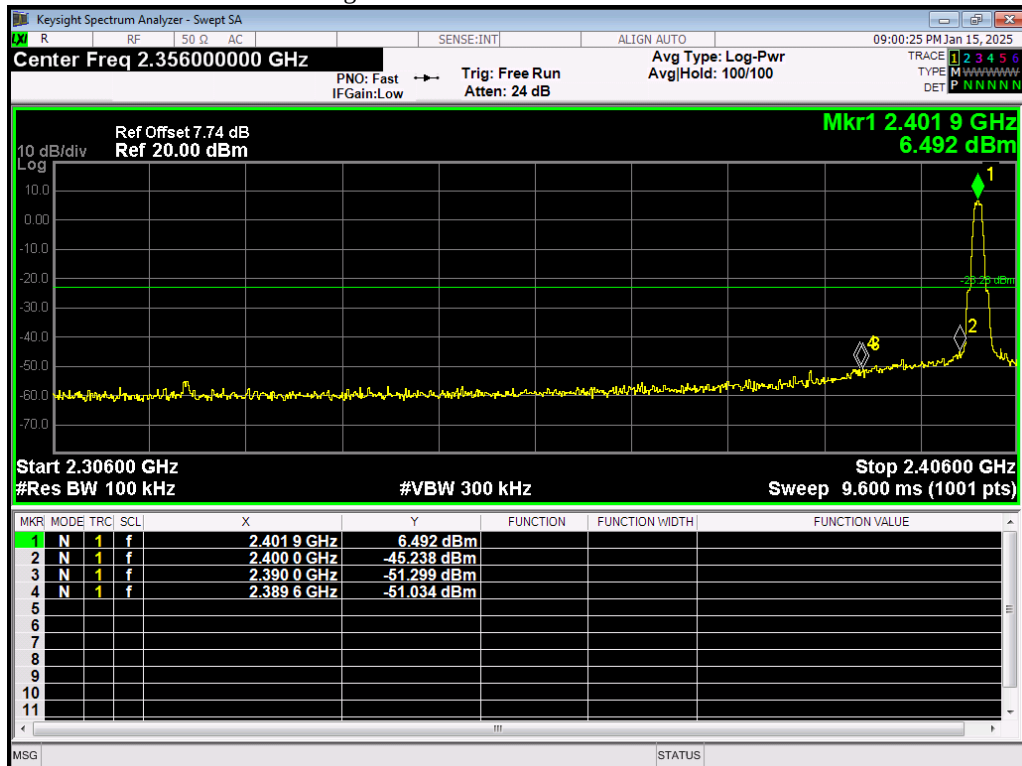
Band Edge NVNT BLE 2402MHz Ant1 Emission
