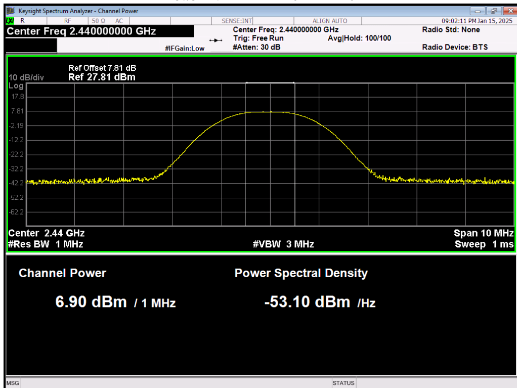
Power NVNT BLE 2440MHz Ant1
