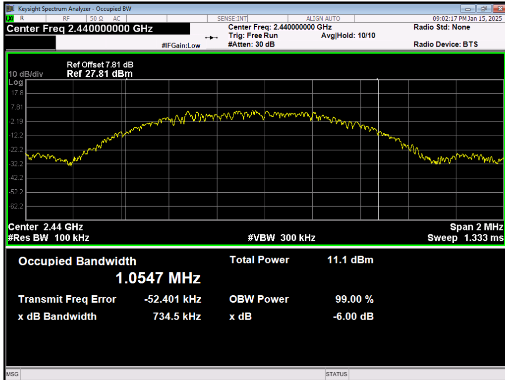
OBW NVNT BLE 2440MHz Ant1
