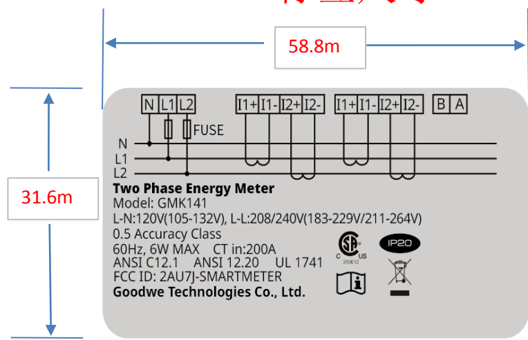
标签尺寸
