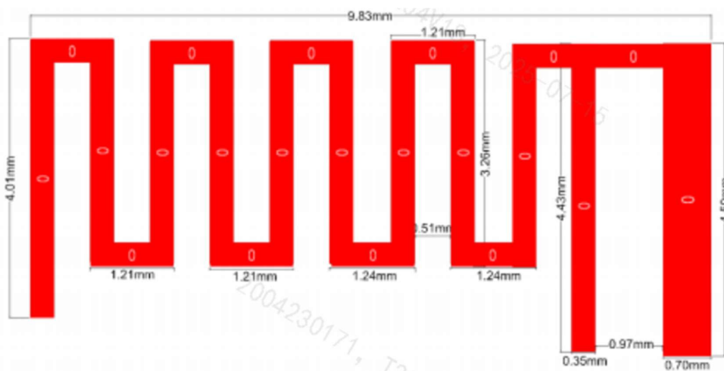
WLT6200 Dimension
