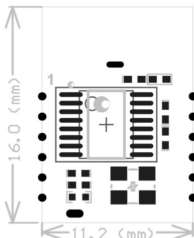
WLT6200 尺寸图
