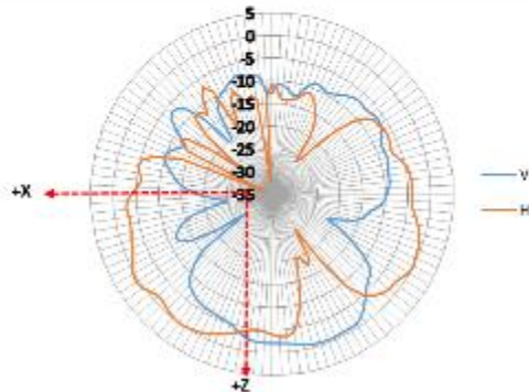
XZ-plane 7125 MHz
