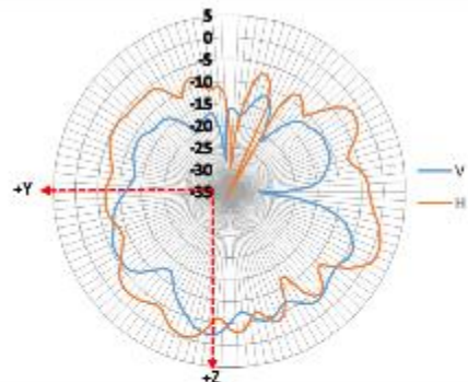
YZ-plane 6875 MHz
