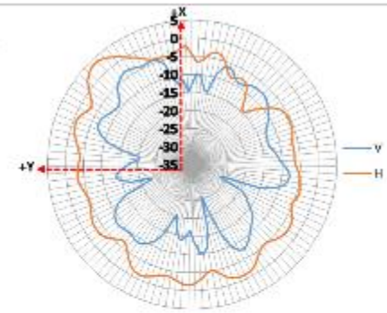
XY-plane 6875 MHz
