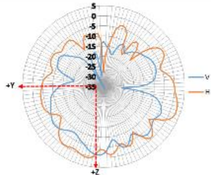
YZ-plane 7125 MHz
