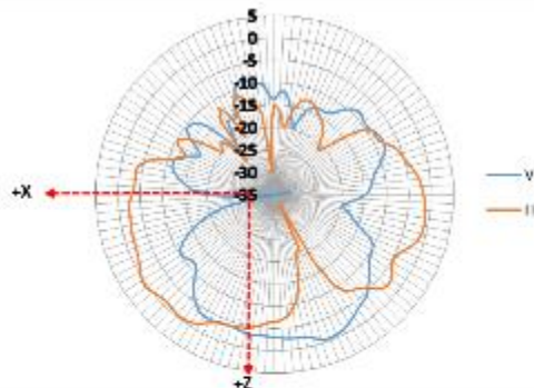
XZ-plane 6875 MHz
