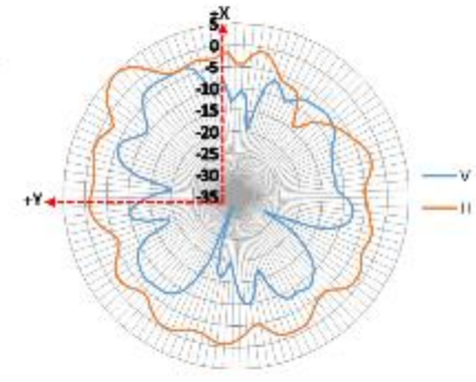
XY-plane 7000 MHz
