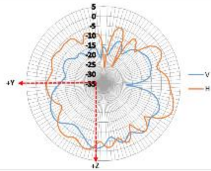
YZ-plane 7000 MHz
