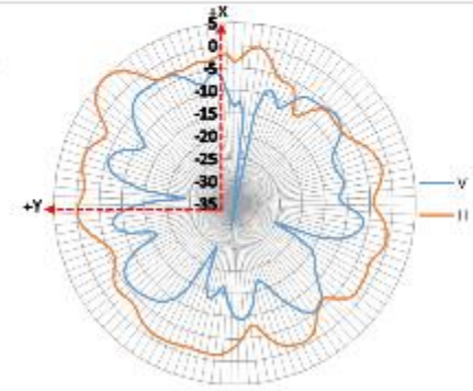
XY-plane 7125 MHz
