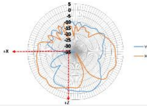
XZ-plane 7000 MHz
