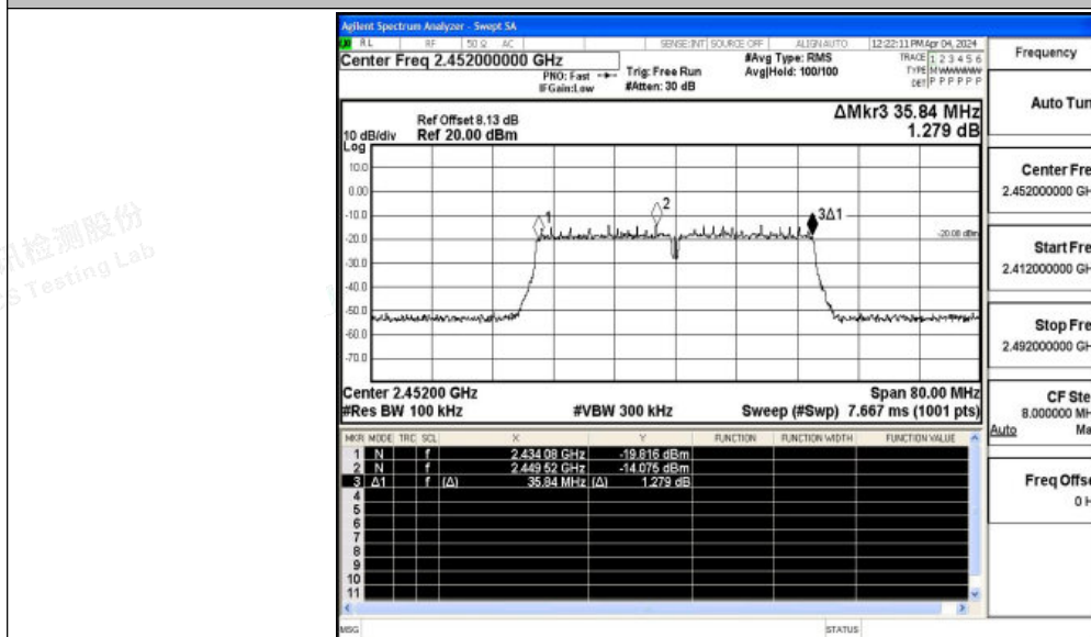
11N40ISO_Ant1_2452
