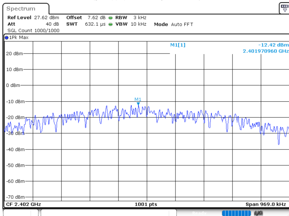
PSD NVNT BLE 2402MHz Ant2
