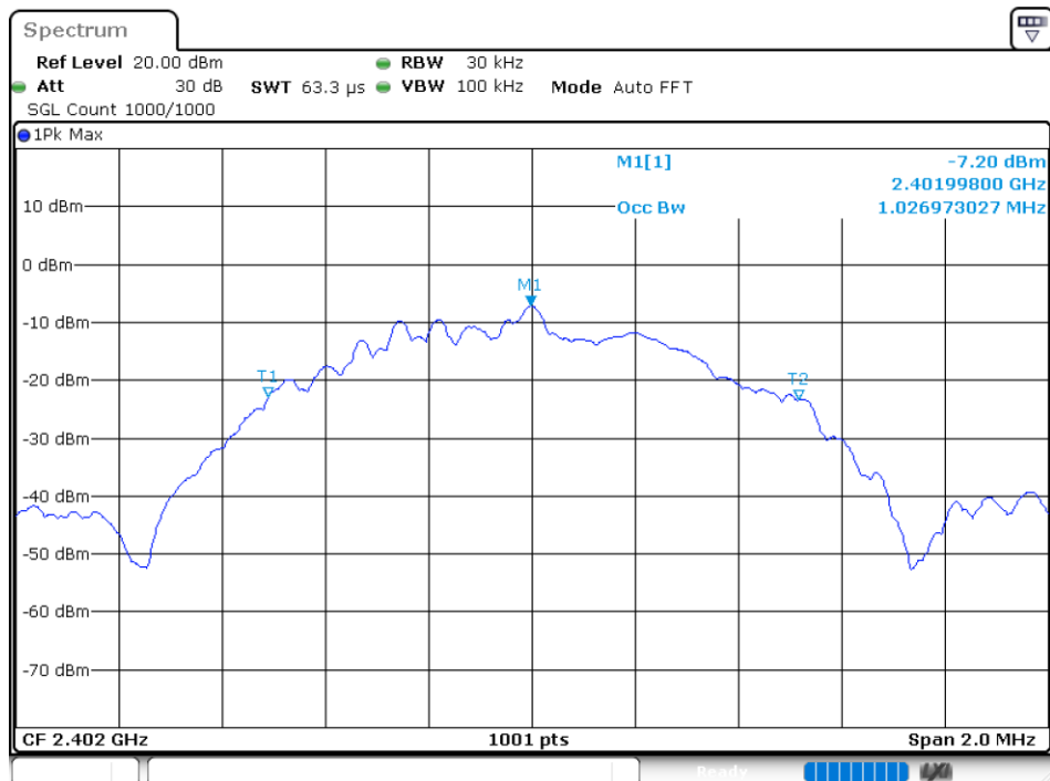
OBW NVNT BLE 2402MHz Ant2
