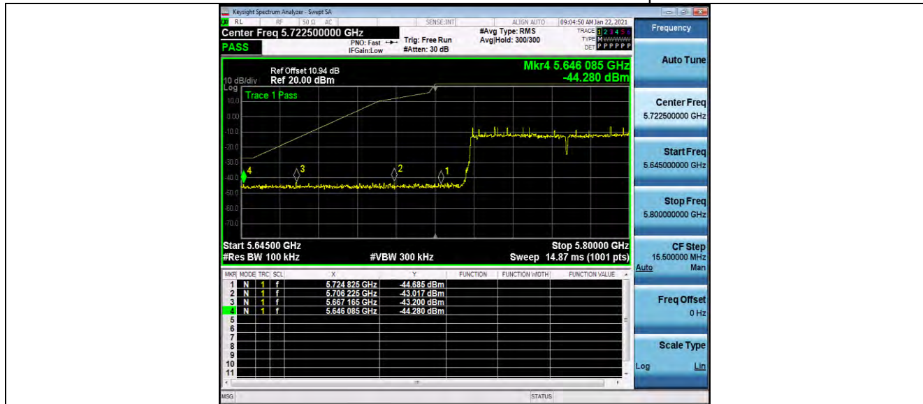
11AC80MIMO_Ant1_Low_5775
