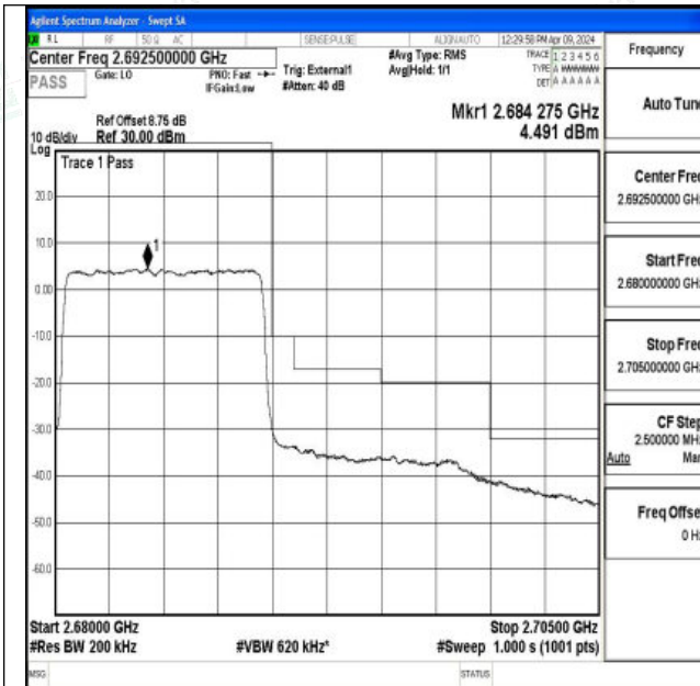
Band41_10MHz_QPSK_41540_50RB#0
