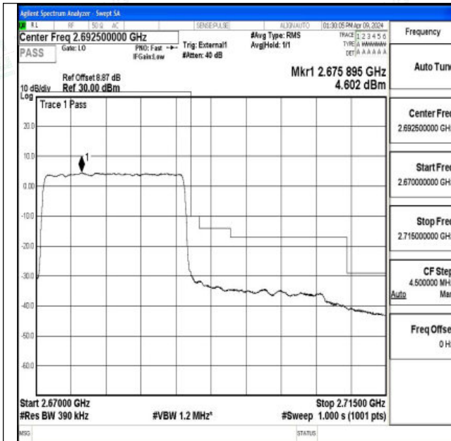
Band41_20MHz_QPSK_41490_100RB#0
