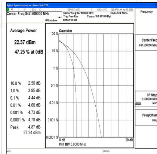
26(824-849)-3MHz-QPSK-27025-1RB#0-PASS
