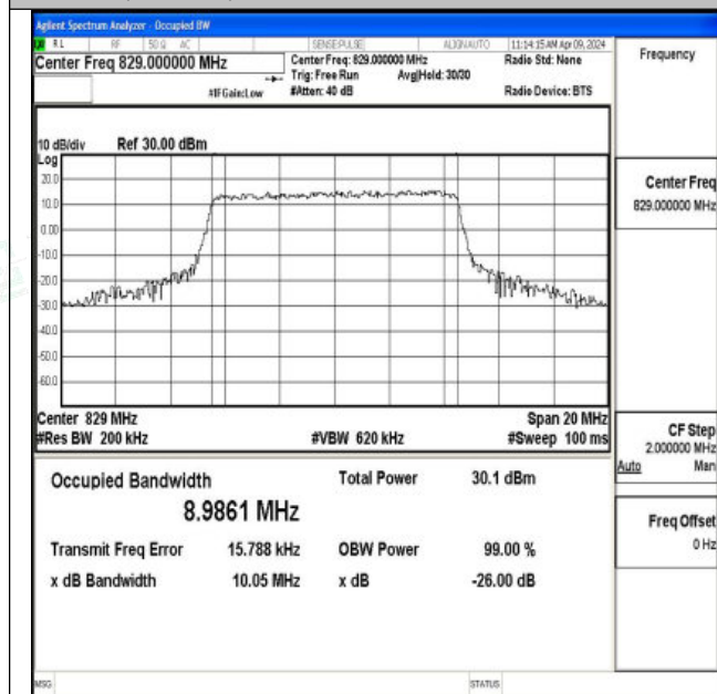
26(824-849)-10MHz-QPSK-26840-50RB#0-PASS
