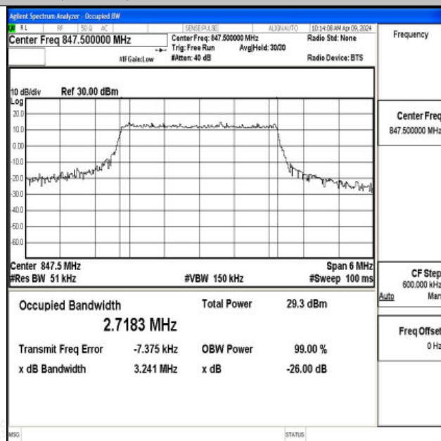
26(824-849)-3MHz-16QAM-27025-15RB#0-PASS
