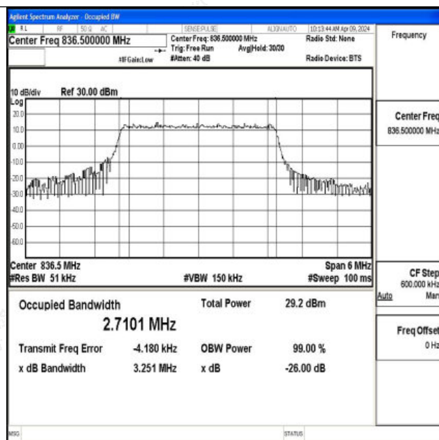
26(824-849)-3MHz-16QAM-26915-15RB#0-PASS
