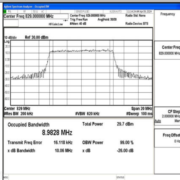
26(824-849)-10MHz-16QAM-26840-50RB#0-PASS
