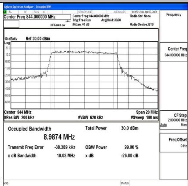
26(824-849)-10MHz-16QAM-26990-50RB#0-PASS
