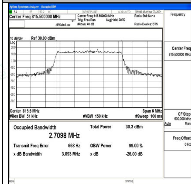
26(814-824)-3MHz-QPSK-26705-15RB#0-PASS
