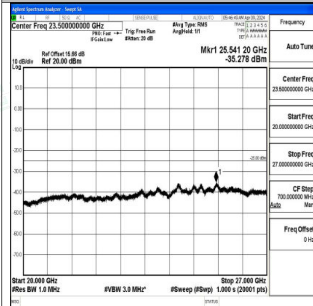
Band7_20MHz_QPSK_20850_1RB#0_20000~27000_20000~27000
