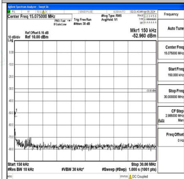
Band4 5MHz 16QAM 20375 1RB#0 0.15~30 0.15~30
