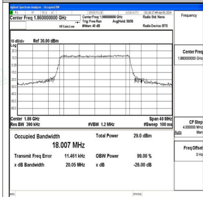
Band2-20MHz-QPSK-18700-100RB#0-PASS
