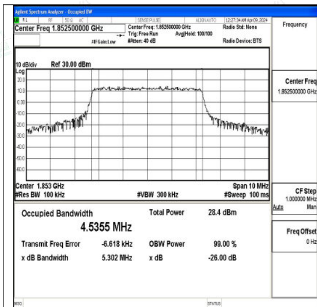
Band2-5MHz-QPSK-18625-25RB#0-PASS
