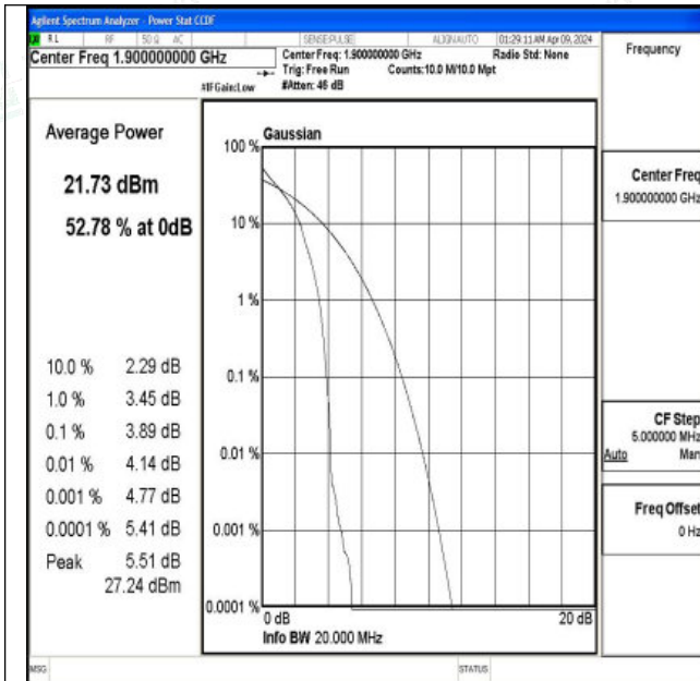
Band2-20MHz-QPSK-19100-1RB#0-PASS
