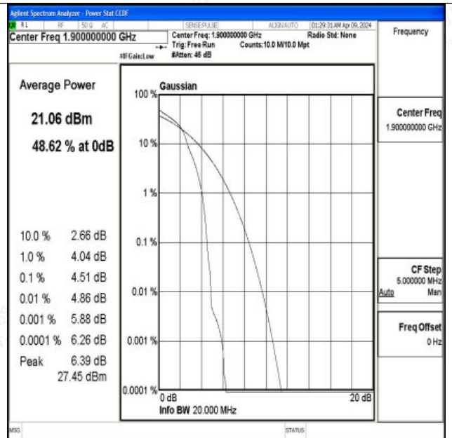
Band2-20MHz-16QAM-19100-1RB#0-PASS
