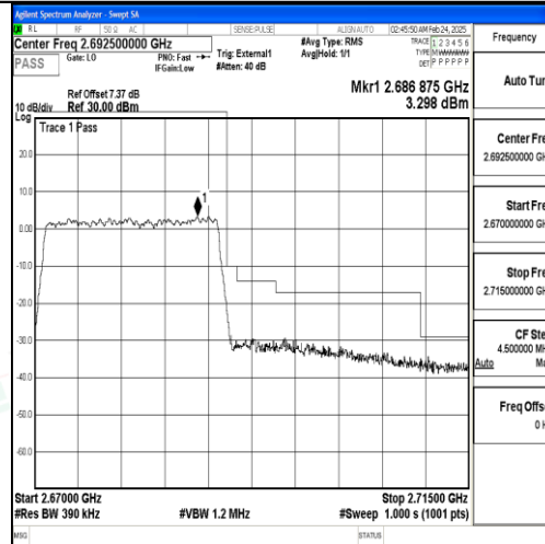
Band41_20MHz_QPSK_41490_100RB#0
