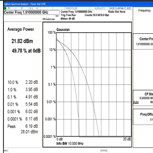
Band25-10MHz-QPSK-26640-50RB#0-PASS
