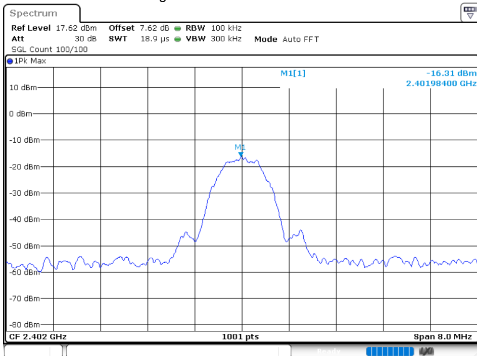
Band Edge NVNT ANT+ 2402MHz Ant1 Ref
