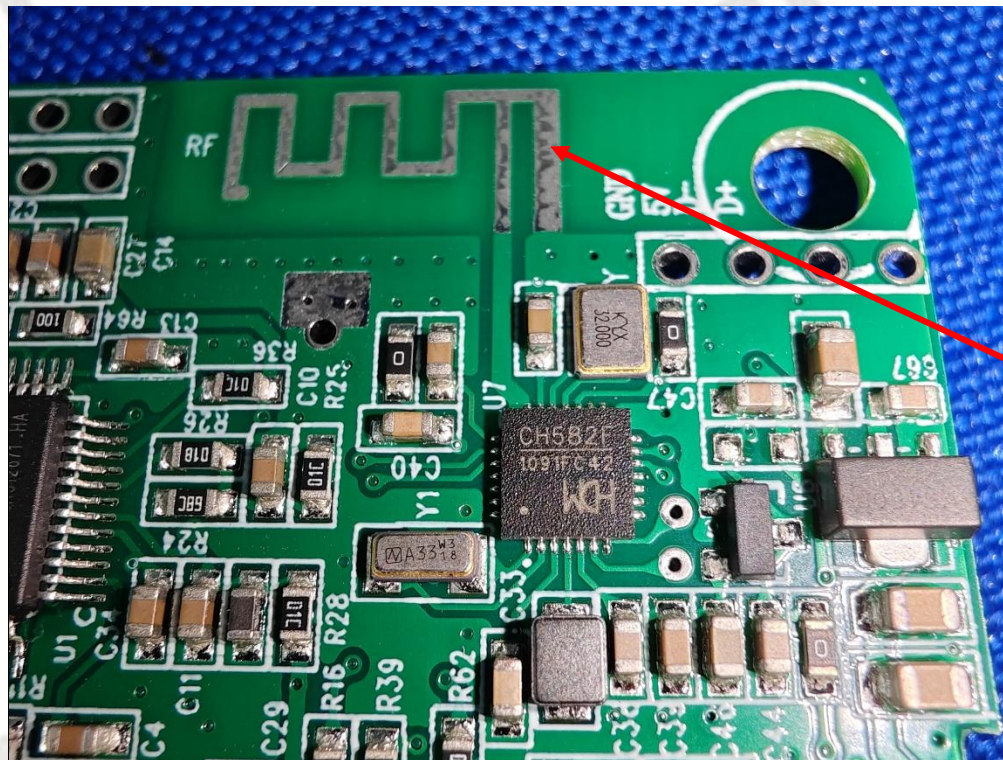
BLE Antenna
