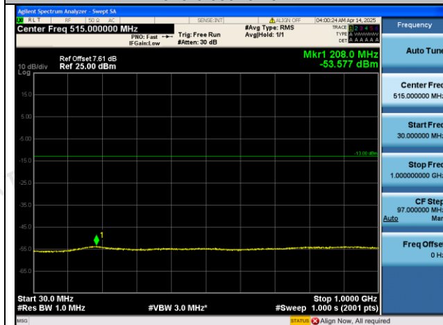
Band4-1513-30~1000MHz-PASS
