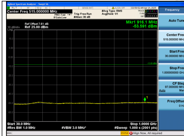
Band4-1413-30~1000MHz-PASS
