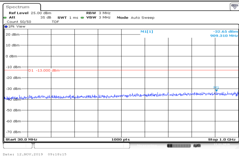
Band4-10MHz-QPSK-20000-50RB#0-Range3:30~1000MHz
