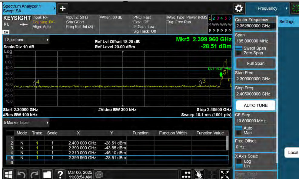
BLE 2M-Ant1-2402-PASS
