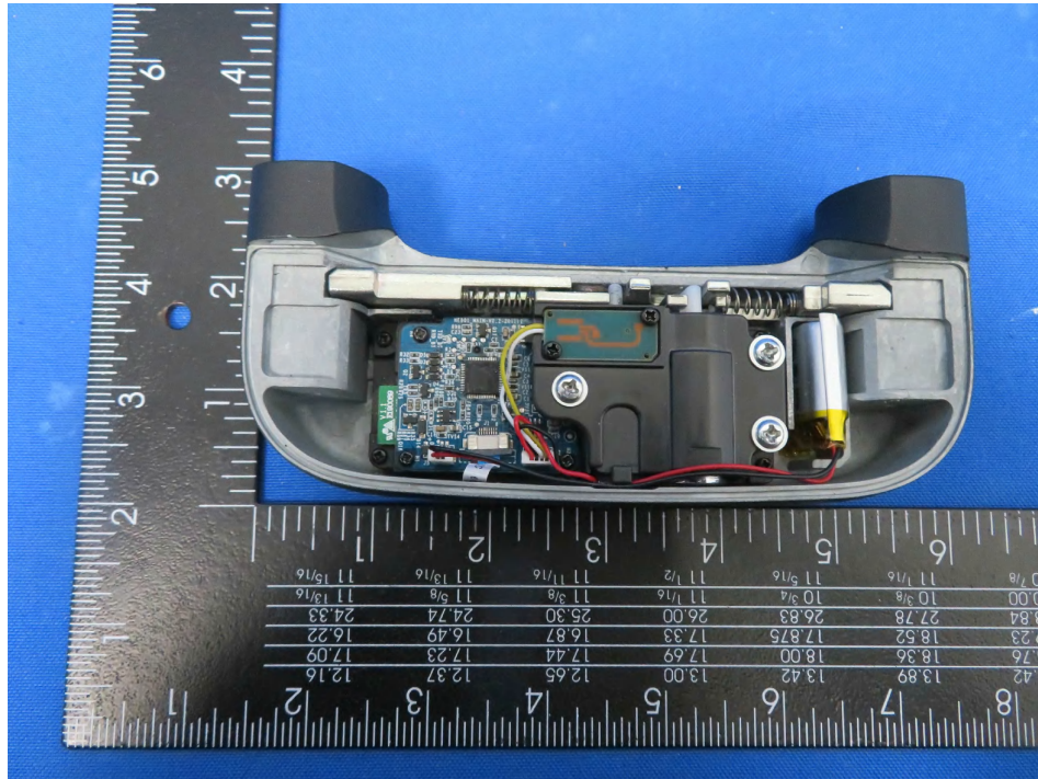
(3) EUT Photo
