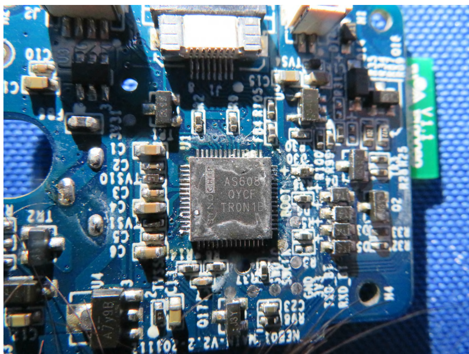
(8) EUT Photo
