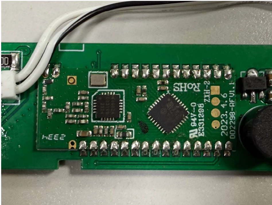
RF Module
