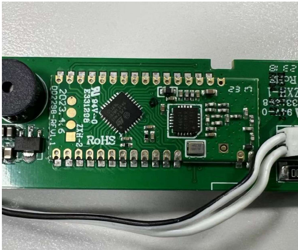
RF Module
