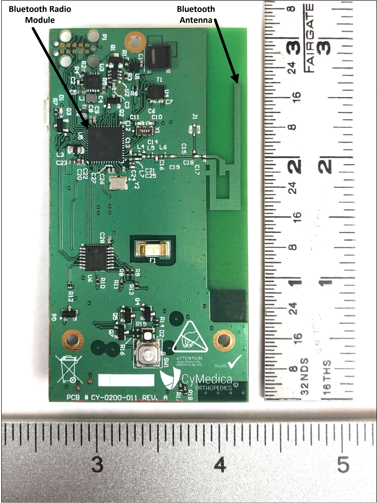
e-vive II Controller PCBA - TOP
