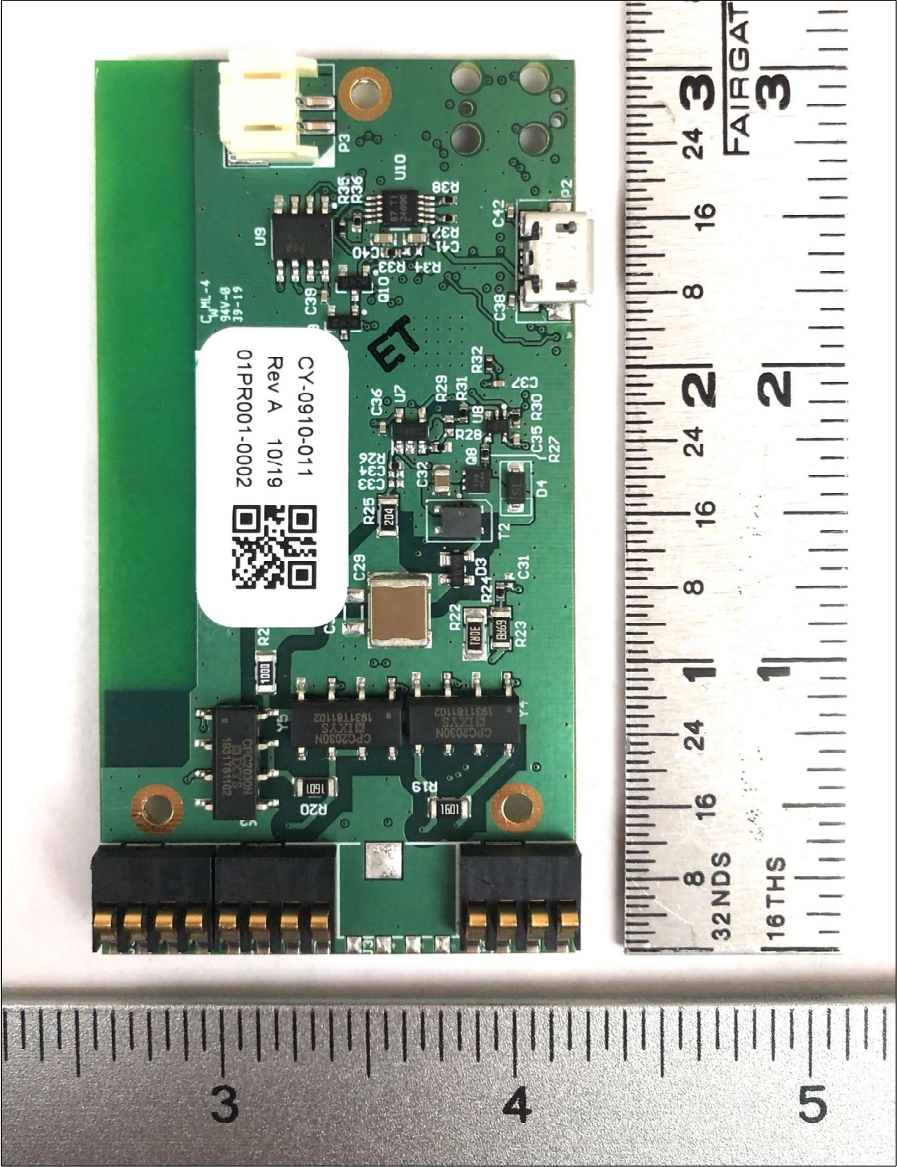
e-vive II Controller PCBA - BOTTOM
