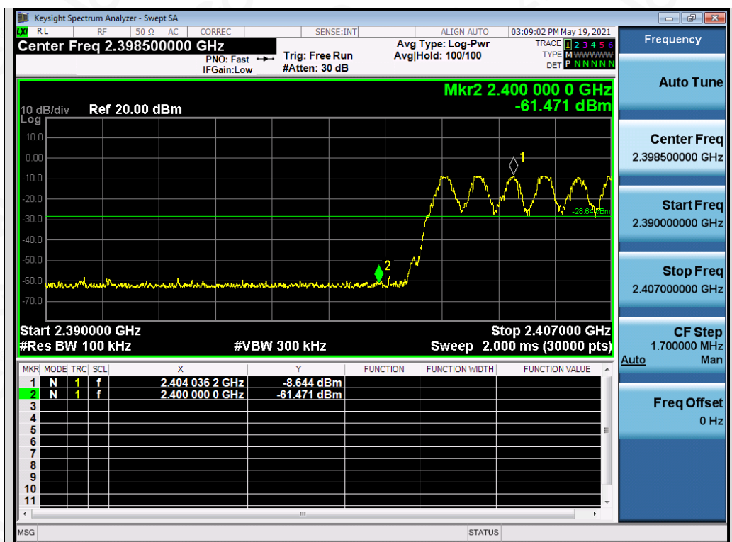
Test_Graph_BR_HOP_ANT2_NA_1Mbps_Lower Band Edge Emissions
