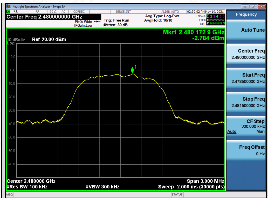
Test_Graph_EDR_ANT2_2480_2Mbps_Reference Level
