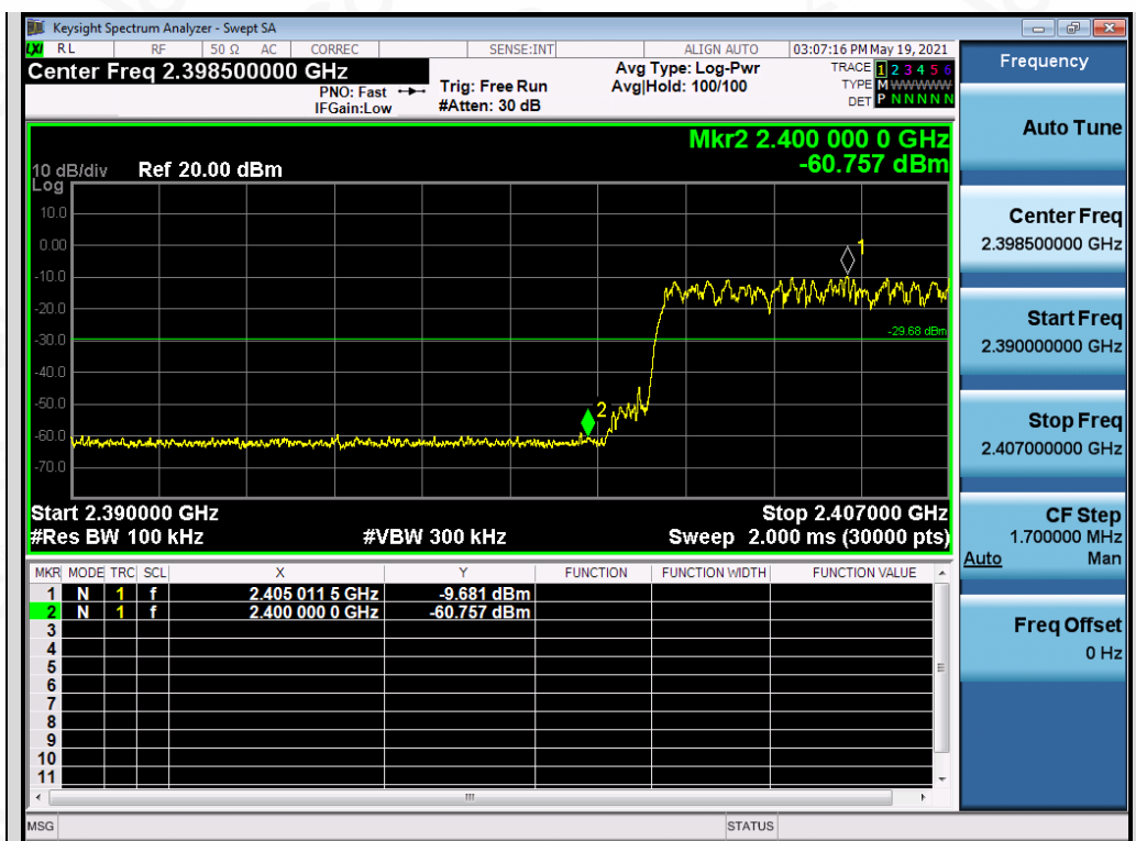
Test_Graph_EDR_HOP_ANT2_NA_3Mbps_Lower Band Edge Emissions
