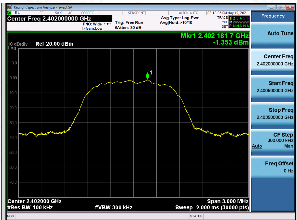
Test_Graph_EDR_ANT2_2402_2Mbps_Reference Level
