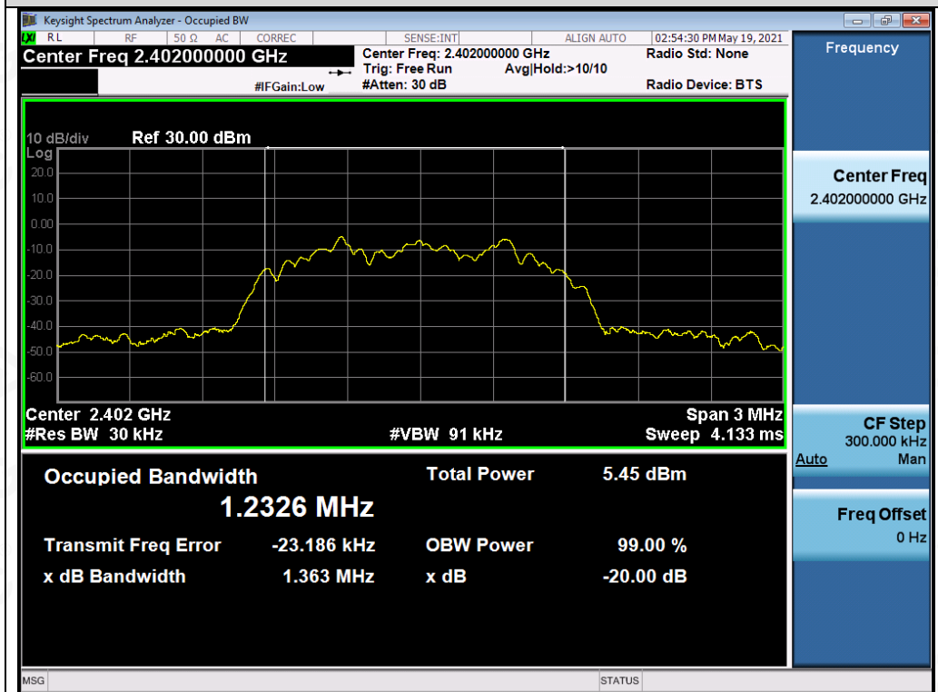
Test_Graph_EDR_ANT2_2402_3Mbps_OBW
