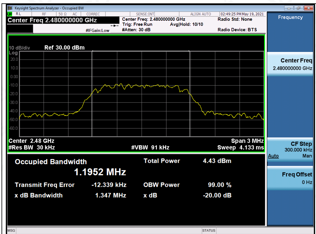
Test_Graph_EDR_ANT2_2480_2Mbps_OBW
