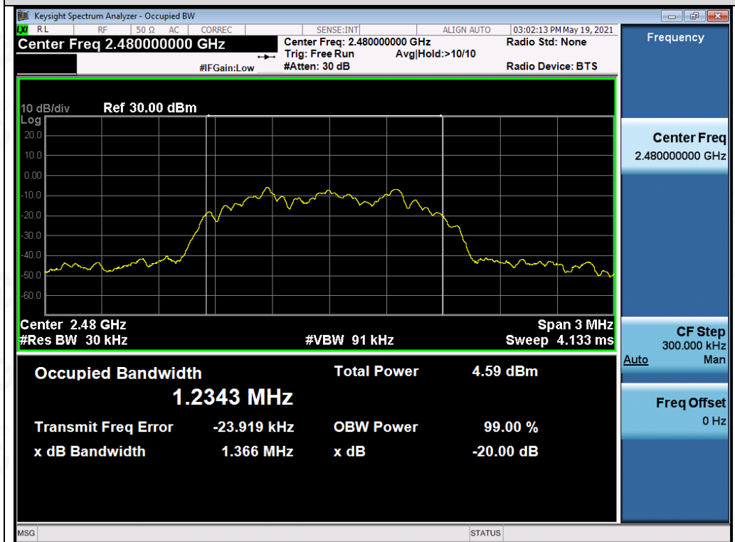
Test_Graph_EDR_ANT2_2480_3Mbps_OBW
