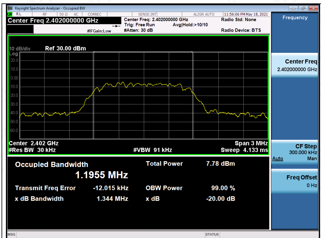
Test_Graph_EDR_ANT2_2402_2Mbps_OBW
