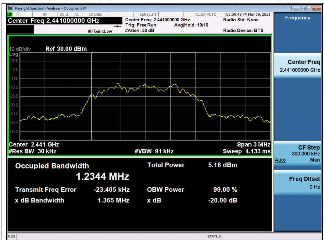
Test_Graph_EDR_ANT2_2441_3Mbps_OBW
