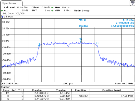
802.11n20_2437MHz 17.560MHz
