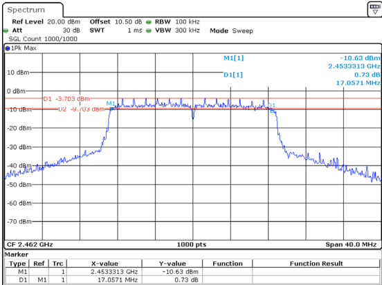
802.11n20_2462MHz 17.057MHz
