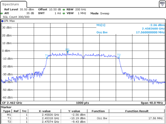
802.11n20_2462MHz 17.560MHz
