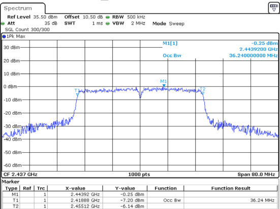
802.11n40_2437MHz 36.240MHz
