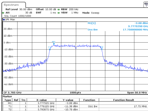
802.11ac20_5785MHz 17.750MHz
