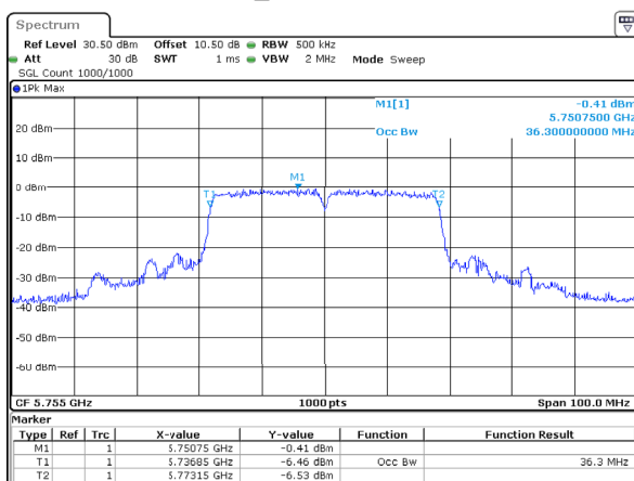
802.11ac40_5755MHz 36.300MHz
