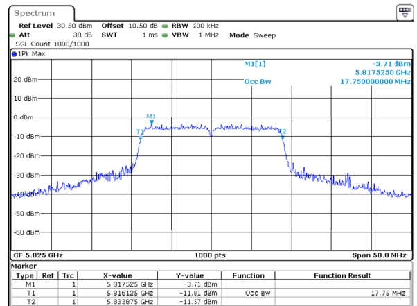
802.11ac20_5825MHz 17.750MHz
