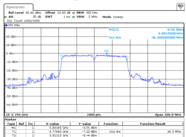
802.11ac40_5795MHz 36.300MHz
